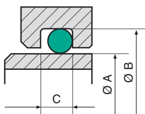
Tenuta stelo Rod application
