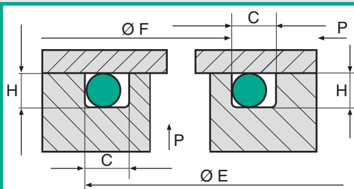
Pressione interna Internal pression Pressione esterna External pression
